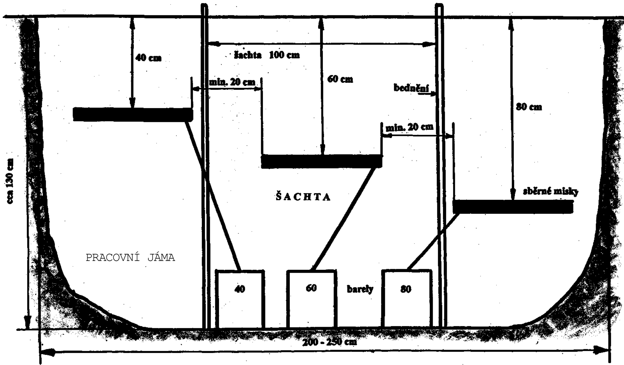
Příloha č.3: Čelní průřez lyzimetru
